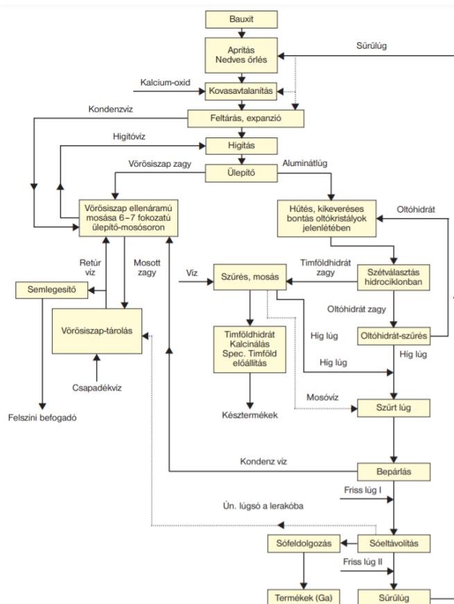
SEQ ábra \* ARABIC 2. ábra: A Bayer-technológia struktúrája. Forrás: Magyar kémikusok lapja LXVI./1. 3. p.
